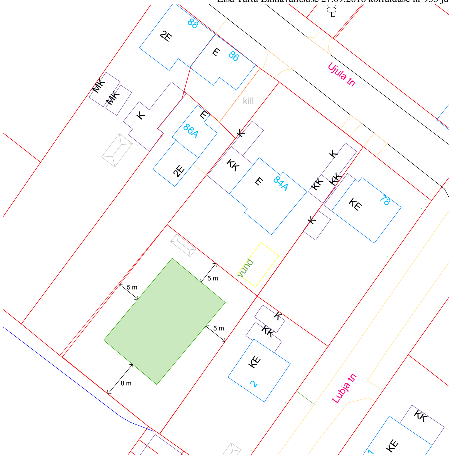
Lisa 1. Ehitusala skeem. Ujula tn 84b PTH-16-155
